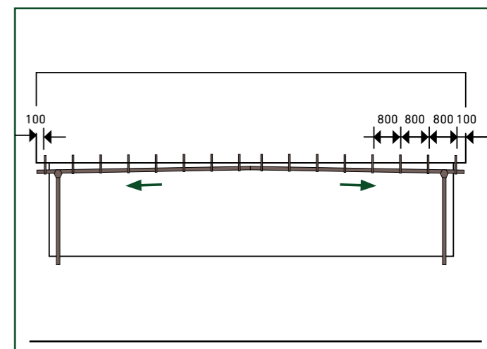
Fig. 2 La lungimi de streășină mai mari de 10 m, se instalează 2 sau mai multe burlane (în funcție de lungime)
