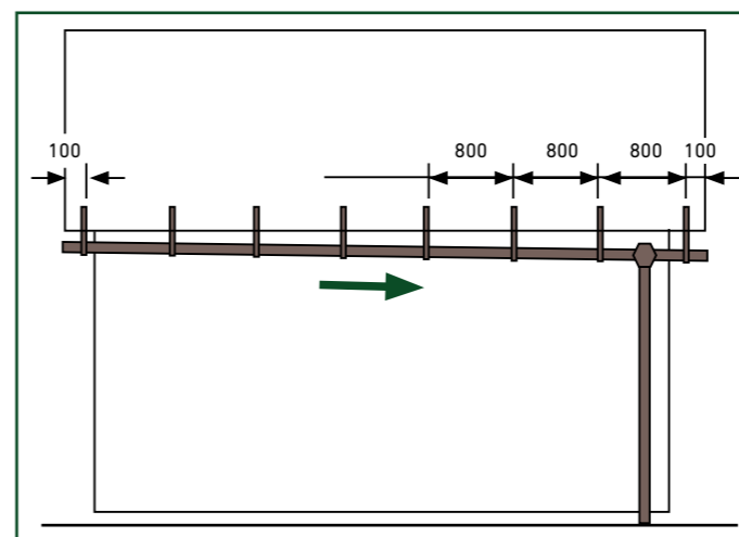
Fig. 1 Pentru lungime streășină de până în 10 m, se instalează un burlan
