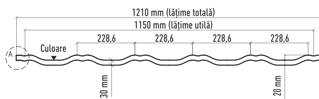
Secțiune transversală
