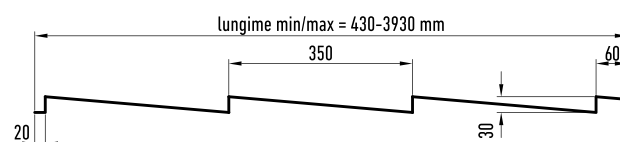
Secțiune longitudinală
